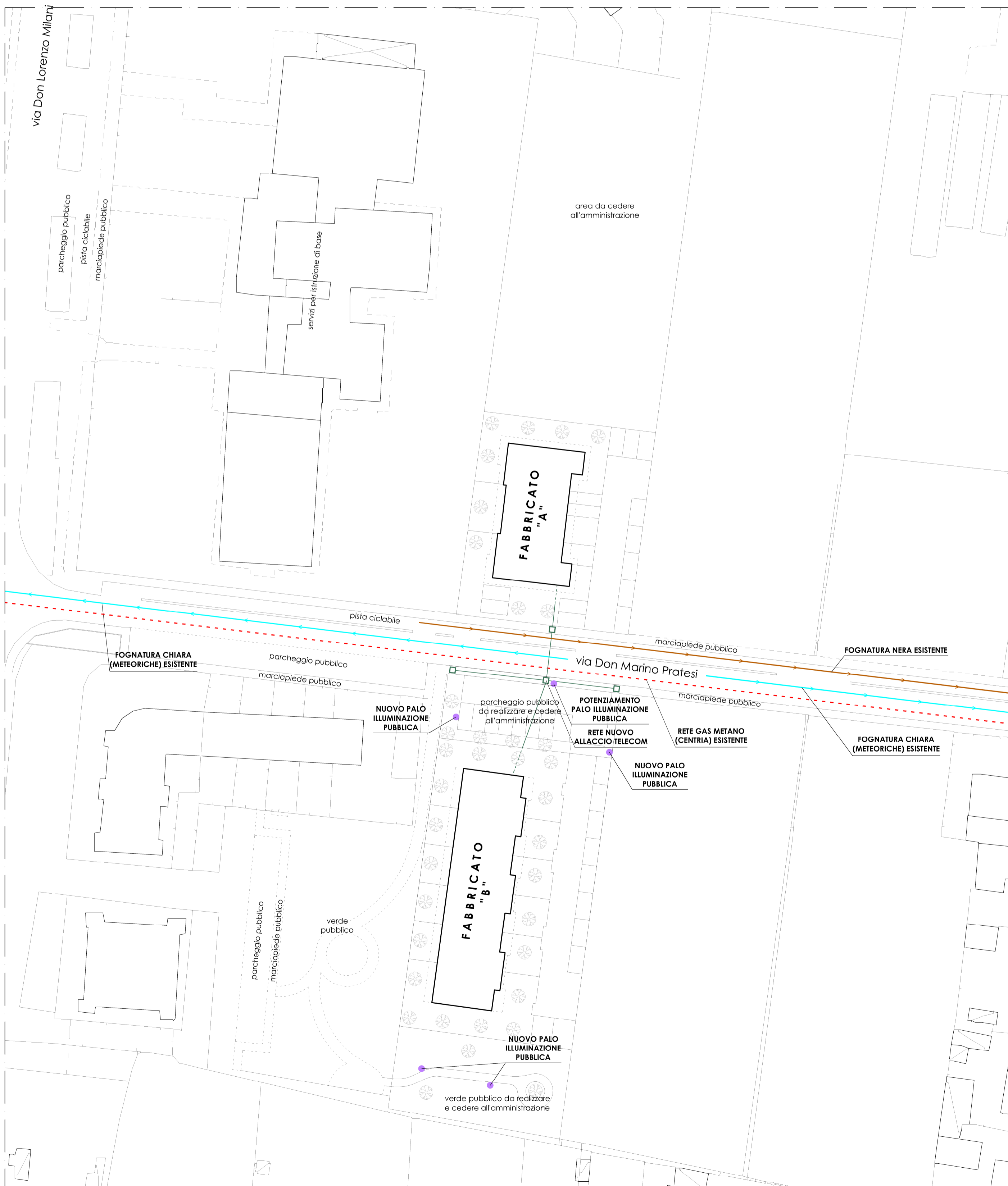
PLANIMETRIA SCHEMA RETI URBANIZZAZIONE - scala 1:500 -
